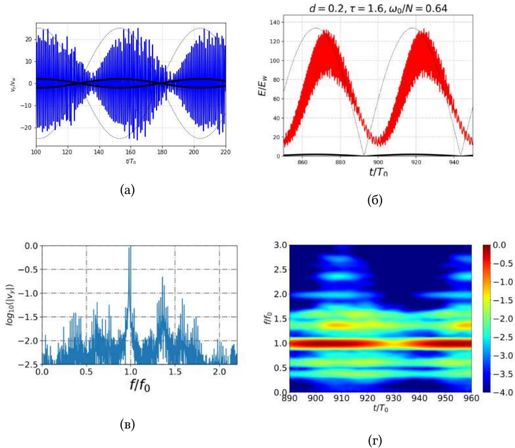
Рис. 6: Вертикальная компонента скорости (а), кинетическая энергия (б), спектр (в) и частотно-временная диаграмма (г) в бигармоническом режиме с амплитудами a = 0.05 \text{ cm/s} и относительной разностью между частотами 0.02. Черной линией на (а) и (б) показана огибающая амплитуды колебаний волнородуктора.
